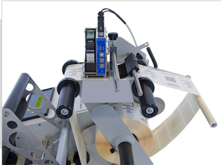
Inkjet marker
