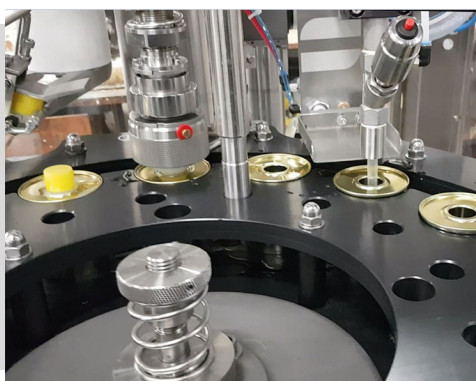
Monobloc 1 tête de remplissage et 1 tête d'enfonçage
